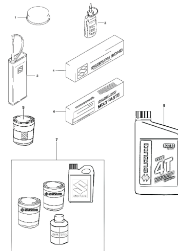
FIG.46 OPTIONAL-2
