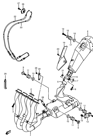
FIG.15 MUFFLER (C-5)
