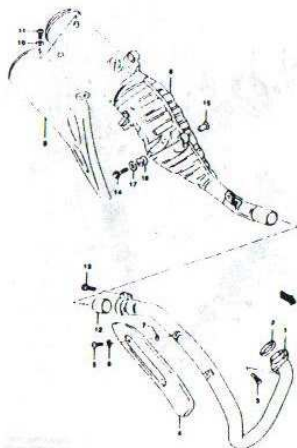
FIG. 12 MUFFLER (C-6)
