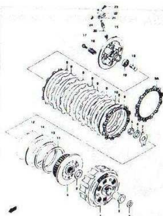
FIG. 17 CLUTCH (C-11)
