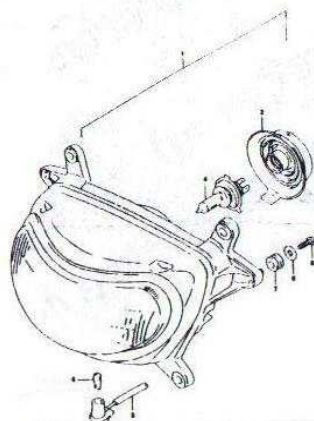
FIG. 25 HEADLAMP (MODEL V/W/X E2,E24) (D-7)
