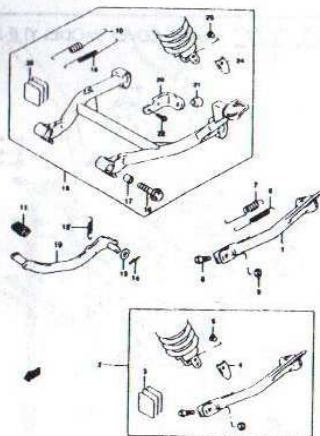
FIG. 32 STAND (E-4)
