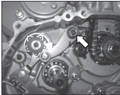
Tuerca patín
